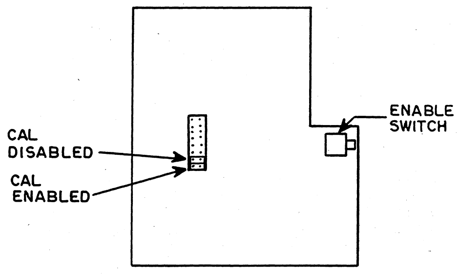
BOTTOM PCB
